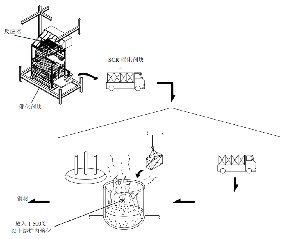
图 C.1 催化剂无害化处理过程
