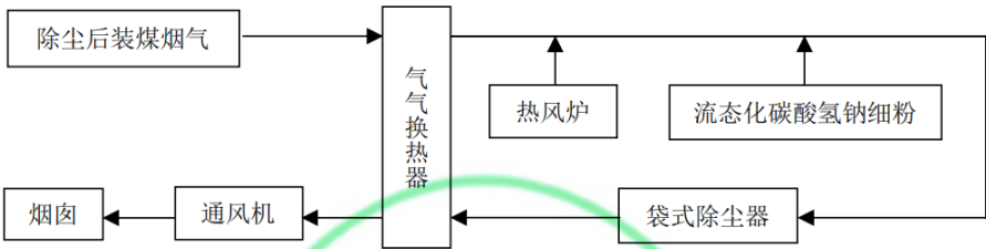
图 3 装煤钠基干法脱硫工艺流程
