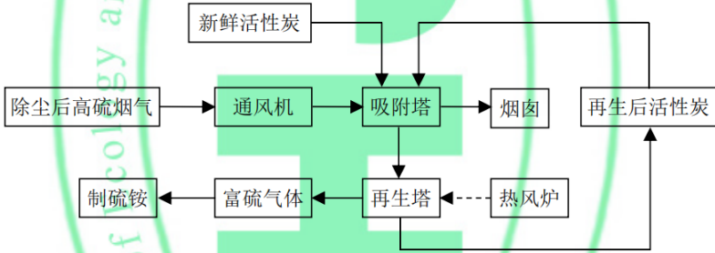
图 17 活性炭（焦）法脱硫工艺流程
