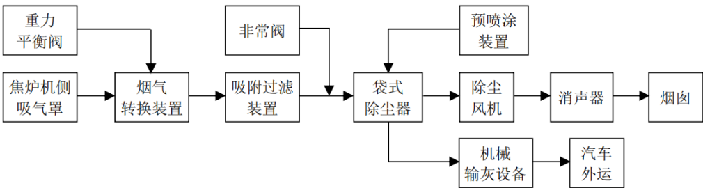
图 8 捣固焦炉机侧除尘地面站工艺流程
