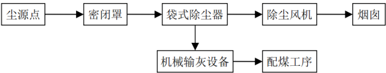
图 1 备煤除尘工艺流程
