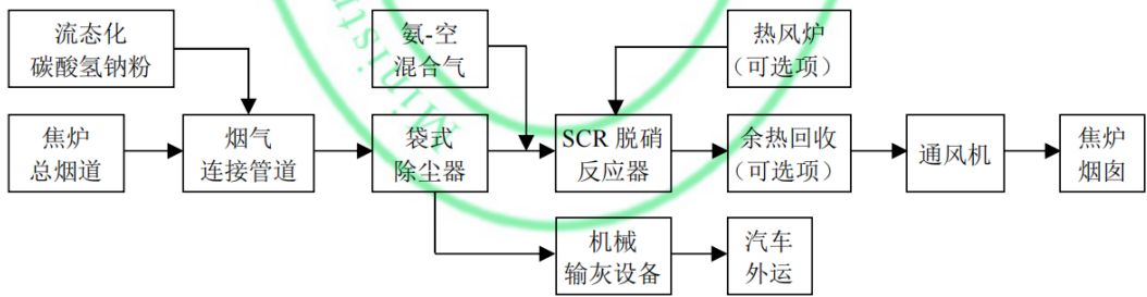
图 9 “钠基干法脱硫+除尘+脱硝”工艺流程
