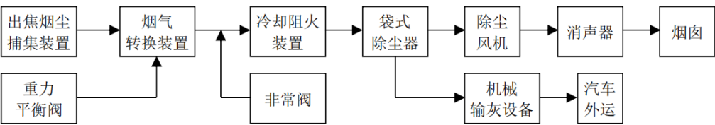
图 6 出焦除尘地面站工艺流程
