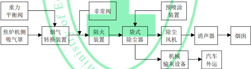
图 7 顶装焦炉机侧除尘地面站工艺流程
