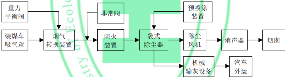
图 2 装煤除尘地面站工艺流程
