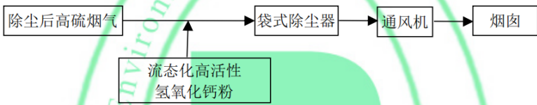
图 16 钙基干法脱硫工艺流程
