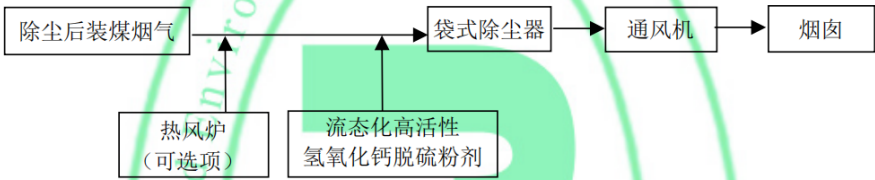
图 4 钙基颗粒床干法脱硫工艺流程
