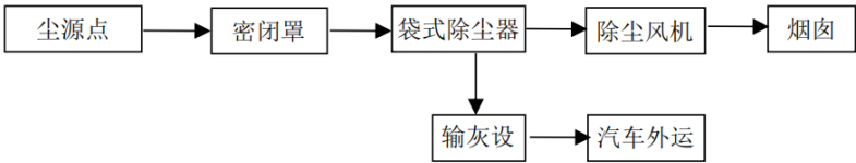
图 18 焦处理除尘工艺流程
