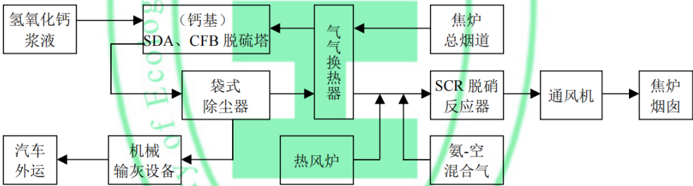
图 12 “钙基半干法脱硫+除尘+脱硝”工艺流程
