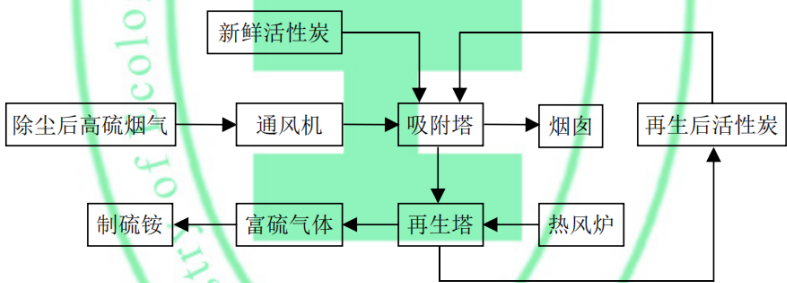
图 5 活性炭（焦）法脱硫工艺流程
