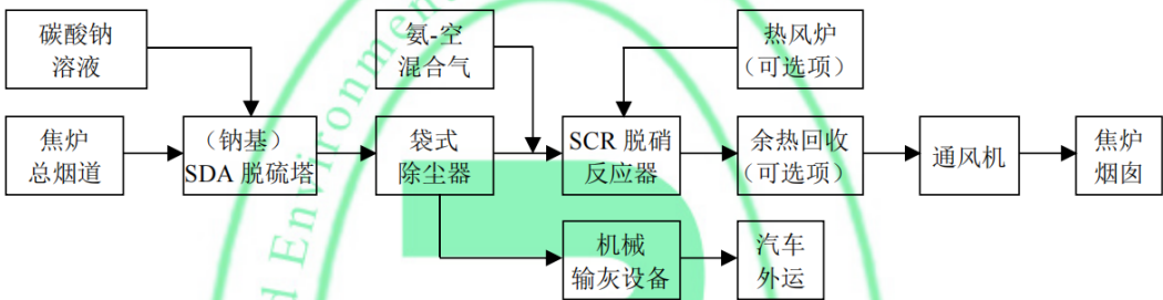
图 11 “钠基半干法脱硫+除尘+脱硝”工艺流程
